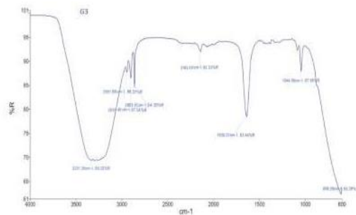
Fig.11: FTIR spectra of SLN gel G3
